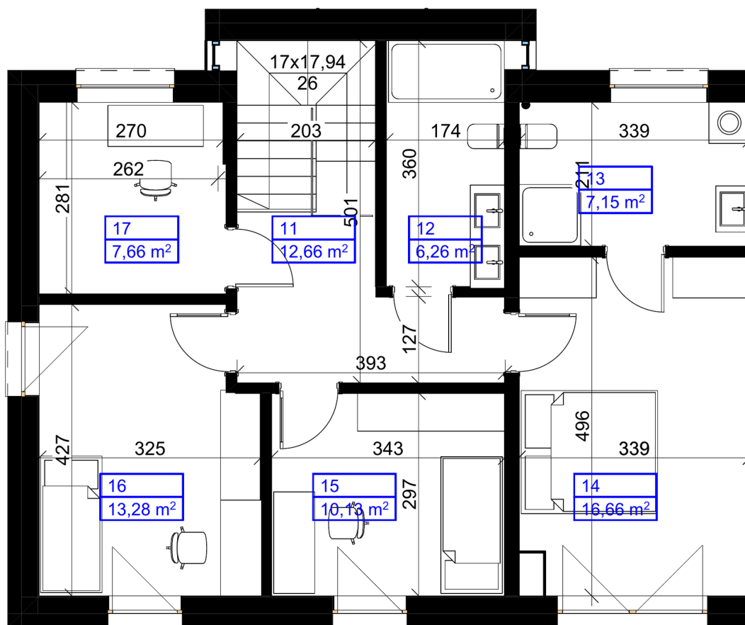
Rzut 2D z wymiarami — układ segmentu 38A
