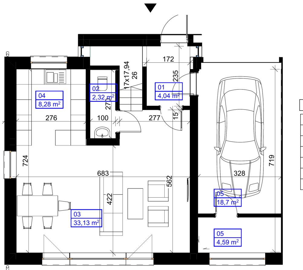
Rzut 2D z wymiarami — układ segmentu 38A
