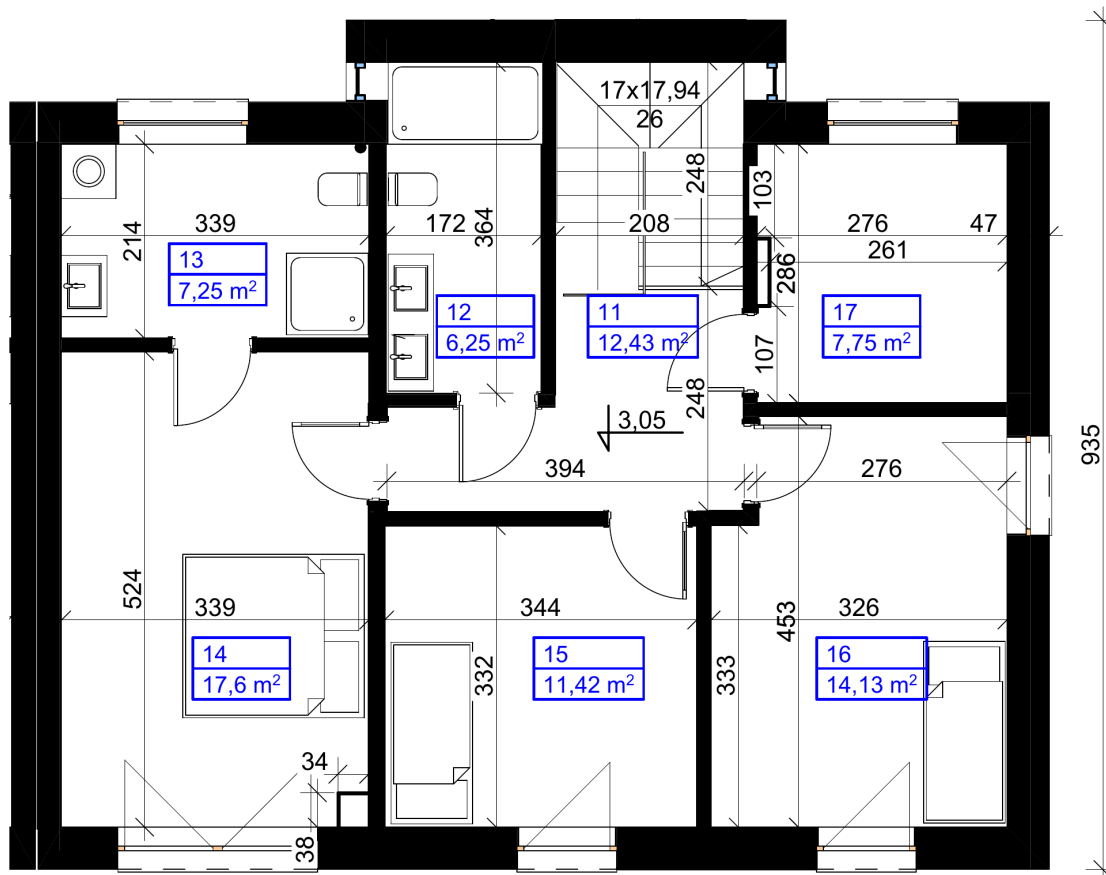
Rzut 2D z wymiarami — układ segmentu 40B
